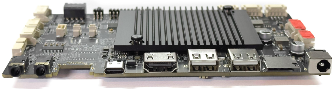
正面图
